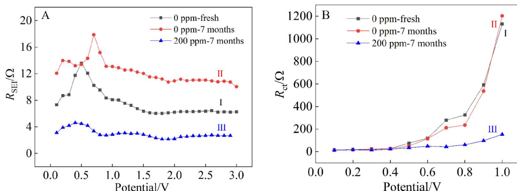
图 6 石墨电极在新鲜的基础电解液、贮存 6 个月后的基础电解液和贮存 6 个月含 200 ppm 白藜芦醇的电解液中(A) R_{SEI} 和(B) R_{ct} 随电极电位的变化。(网络版彩图)
