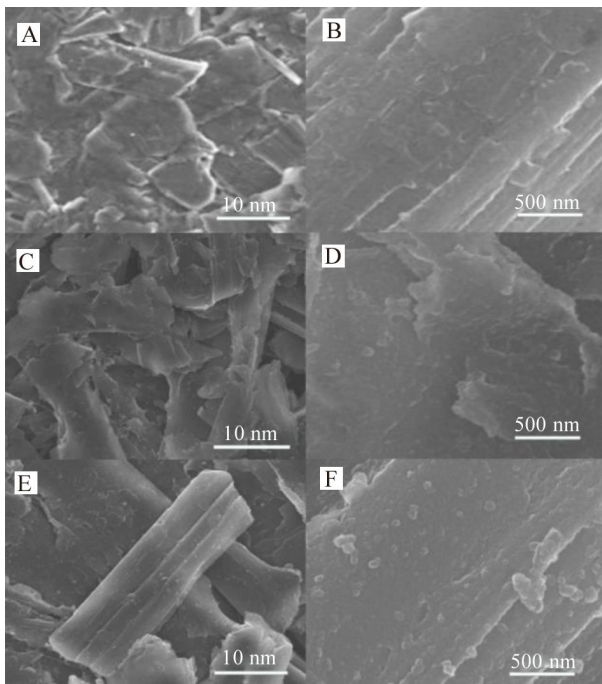
图 7 石墨电极在(A)-(B)新鲜的基础电解液、(C)-(D)贮存 6 个月后的基础电解液和(E)-(F)贮存 6 个月后含有 200 ppm 白藜芦醇的基础电解液中经历充放电循环 10 周后的 SEM 图像。
