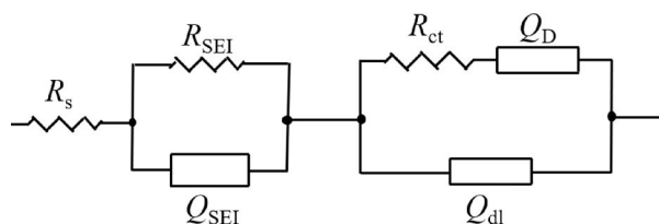
图 5 石墨电极首次放电过程的等效电路图
