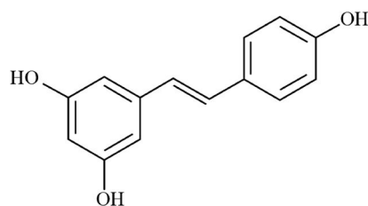
图 1 白藜芦醇的结构式
