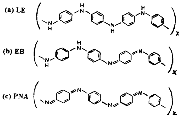
图6 不同氧化态的聚苯胺的三种构型 Fig. 6 (a) Leucoemeraldine, (b) Emeraldine, and (c) Pernigraniline base formsof polyaniline
