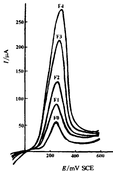
图 2 不同载荷条件下 18/8 不锈钢在 \text{Na}_2\text{S}_2\text{O}_3 + 0.1\% HCl 溶液中的阳极极化行为的比较
