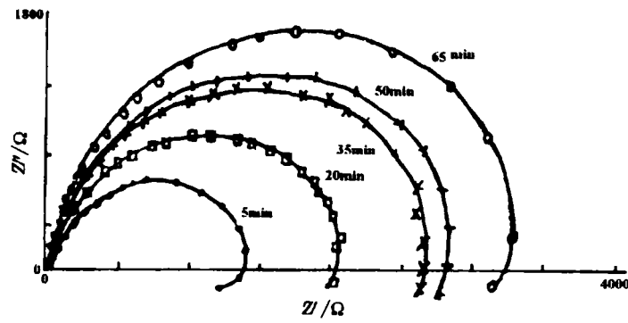
图6 载荷条件下18/8 不锈钢在2 mmol/L Na 2 S 2 O 3 +0.1% HCl 溶液中交流阻抗频谱随时间的变化
