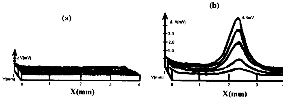
图7 载荷条件下18/8 不锈钢在2 mmol/L Na 2 S 2 O 3 +0.1% HCl 溶液中当控制不同电位时表面二维方向电流密度分布的测量
