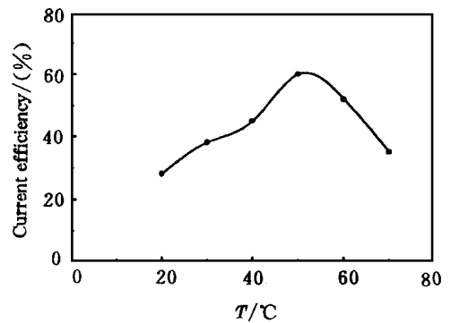
图3 温度对顺丁烯二酸的阴极间接环氧化反应电流效率的影响
