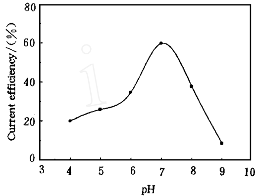
图2 pH值对顺丁烯二酸阴极间接环氧化反应电流效率的影响
