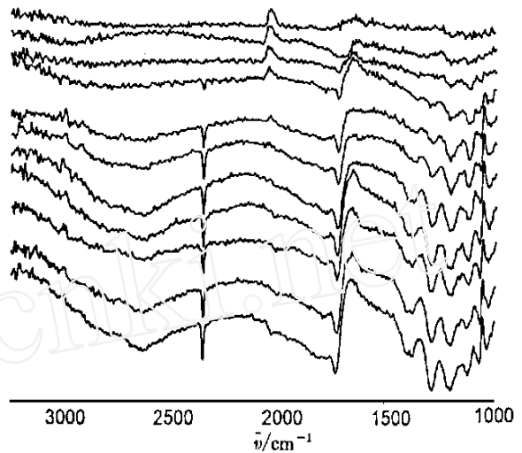
图 2 E_R = -0.25 \text{ V} , E_S 从 0.0 \text{ V} 升高到 1.0 \text{ V} 的原位 FTIR 反射光谱
