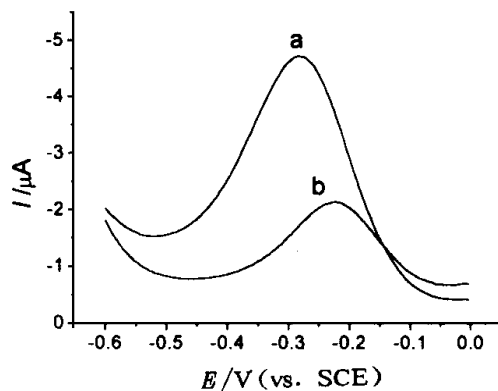
图5 吸附硫堇在 DNA/ PDPA 电极上的微分脉冲伏安图
