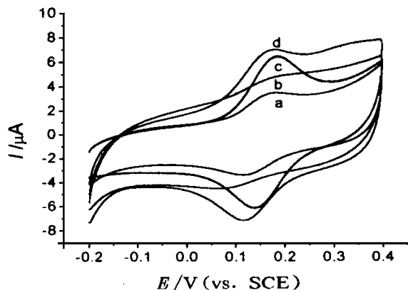
图4 [\text{Co}(\text{phen})_3]^{3+/2+} 在不同电极上的循环伏安图
