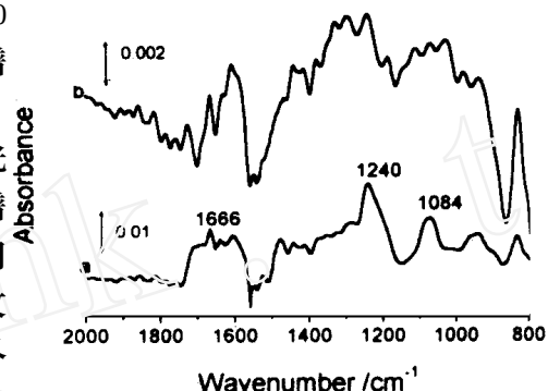
图 1 dsDNA/ PDDA/ Au (a) 和 ssDNA/ PDDA/ Au 的红外漫反射谱图
