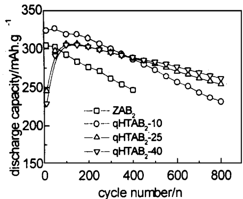
图3 不同制备方法的 Zr_{0.9}Ti_{0.1}(Ni,Co,Mn,V)_{2.1} 贮氢合金在电流为 300\text{ mA}\cdot\text{g}^{-1} 下的循环稳定性
