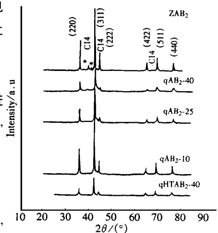
图 1 不同方法制备的各种 Zr_{0.9}Ti_{0.1}(Ni,Co,Mn,V)_{2.1} 合金的 XRD 衍射图
