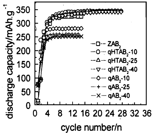
图 2 不同方法制备的的各种的 Zr 0.9 Ti 0.1 (Ni, Co, Mn, V) 2.1 贮氢合金在 60 mA.g -1 电流密度下放电容量与循环次数的关系
