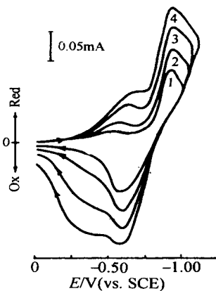
图2 \text{Cd}(p\text{-CH}_3\text{C}_6\text{H}_4\text{SO}_3)_2 ( 0.0086 \text{ mol} \cdot \text{L}^{-1} ) 在 0.05 \text{ mol} \cdot \text{L}^{-1} TBA P+DM SO 溶液中于Pt电极( 0.096 \text{ cm}^2 )的循环伏安曲线 301 K
