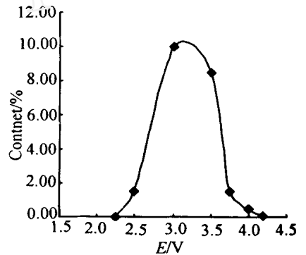
图3 聚合物锂离子电池不同化成电压下产气总量
