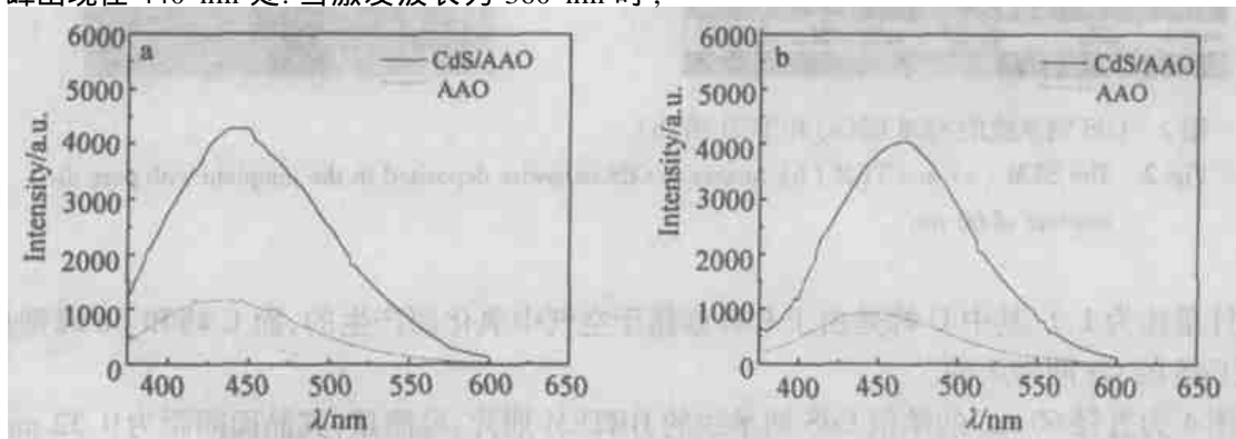
图 6 不同激发波长 ((a) 325 nm 和 (b) 360 nm) 下 CdS/ AAO 纳米线阵列的荧光光谱 Fig.6 Fluorescence spectra of CdS/ AAO and AAO with excitation wavelength of : (a) 325 nm and (b) 360 nm
