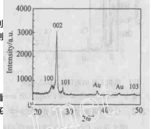
图 1 CdS 纳米线 X 射线衍射图谱
