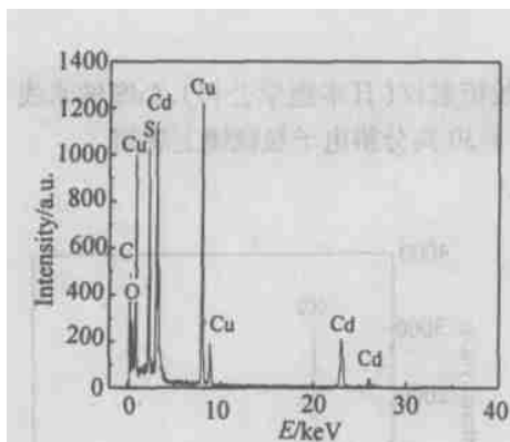
图3 单根 CdS 纳米线的 EDAX 图谱 Fig.3 EDAX spectrum of a single CdS nanowire
