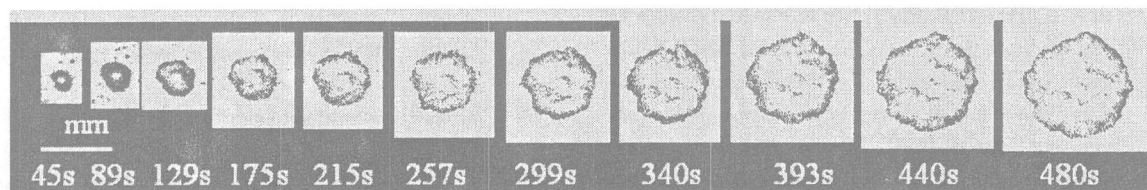
图 6 不同时间针尖点接触电极恒电位 -0.24 \text{ V} (vs SCE) 电解薄层 \text{AgCl} 还原面积变化的光学扫描照片
