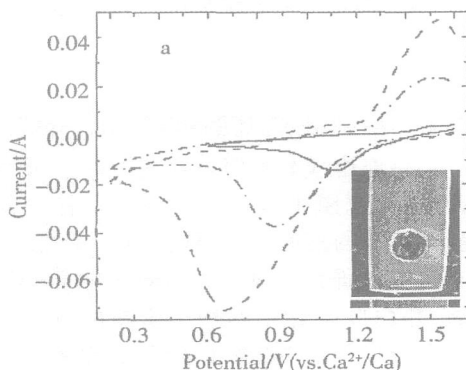
图 5 负载 NiO 粉末的钼腔电极(其 SEM 照片如 a 中插图)于 900 °C \text{CaCl}_2 熔盐中的循环伏安曲线 (a) 及峰电流随扫描速率变化关系 (b) *
