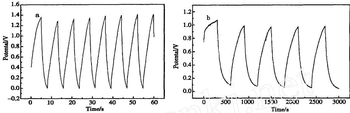
图 3 纳米电容器的充放电曲线 a) STM 针尖 1 nA 5 s, b) Pt 针尖 5 nA 300 s
