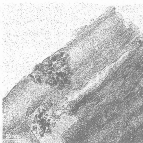
图 2 纳米 PPy/ \text{TiO}_2 /PPy 电容器的 TEM 图
