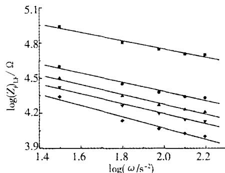
图 8 \log(Z_t)_{LF} 对 \log \omega 关系图
