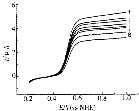
图 5 二茂铁在含有 DNA 溶液中于旋转玻碳电极上的伏安曲线
