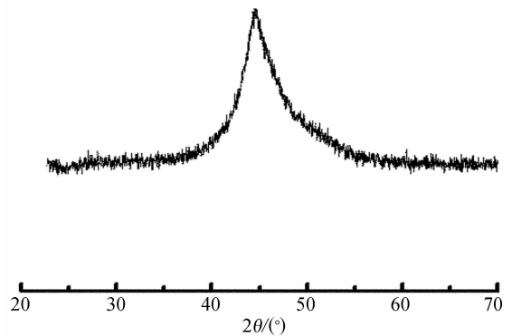
图5 化学镀镍镀层 XRD 谱图
