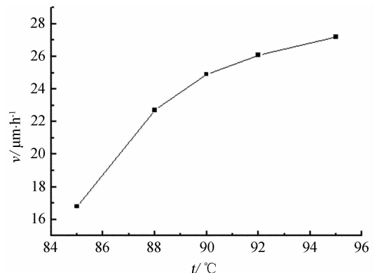
图1 温度对化学镀镍沉积速率的影响
