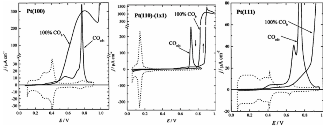
图 3 Pt(100),Pt(110)-1× 1 和 Pt(111)晶面上 CO 在 0.5 mol·L -1 H 2 SO 4 溶液中的溶出伏安曲线 [11]
