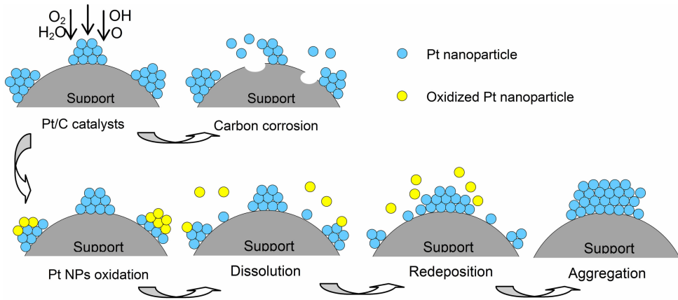
图10 Pt/C纳米催化剂电化学活性表面积降低机理示意图 [26]
