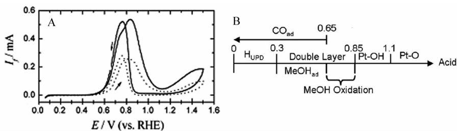
图2 A. 光滑的多晶Pt在0.1 mol·L -1 甲醇 + 0.5 mol·L -1 H 2 SO 4 溶液(虚线)与0.1 mol·L -1 甲醇 + 0.5 mol·L -1 HClO 4 溶液(实线)室温25 °C下的循环伏安曲线, 扫描速率10 mV·s -1 [7]; B. 酸性介质中Pt表面甲醇吸附氧化过程示意图 [8]
