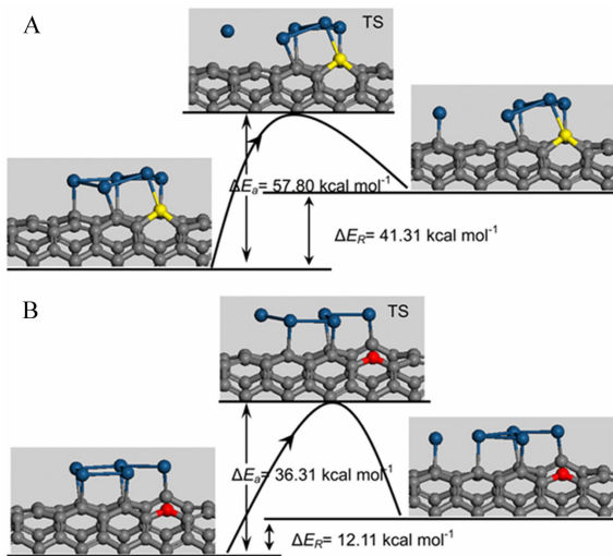
图11 Pt簇分别在SH-SWCNTs (A)和OH-SWCNTs (B)上的迁移反应能 [27]
