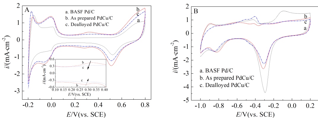
图3 商业化 Pd/C 和去合金化前后 Pd 2 Cu 1 /C 催化剂电极在 0.5 mol·L -1 H 2 SO 4 (A) 和 1 mol·L -1 NaOH(B) 溶液的循环伏安曲线 扫描速率 50 mV·s -1 Fig. 3 Cyclic voltammograms of commercial Pd/C, as prepared Pd-Cu/C and dealloyed Pd-Cu/C in 0.5 mol·L -1 H 2 SO 4 (A) or 1 mol·L -1 NaOH (B) solution at a scan rate of 50 mV·s -1
