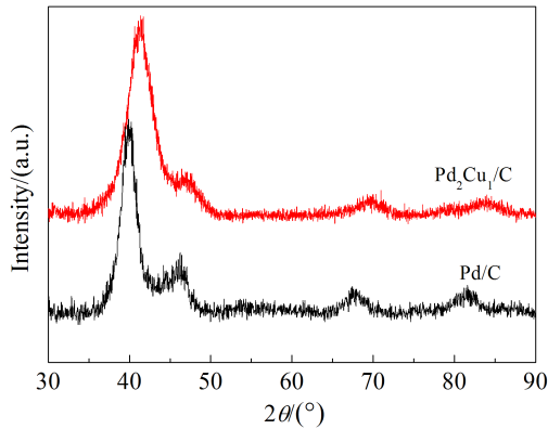
图2 Pd 2 Cu 1 /C 和商业化 Pd/C 样品的 XRD 衍射图 Fig. 2 XRD patterns of as-prepared Pd 2 Cu 1 /C and commercial Pd/C
