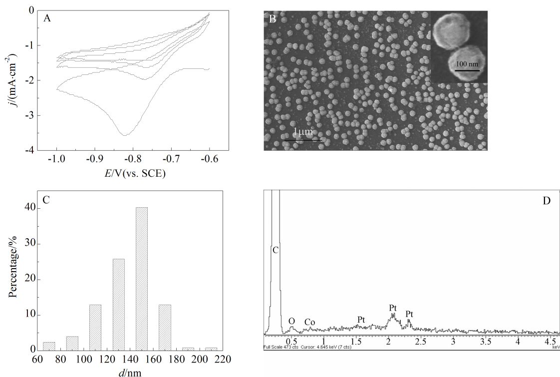
图 1 A. CoPt/GC 循环伏安电沉积曲线, 沉积液 10 \text{ mmol} \cdot \text{L}^{-1} \text{ CoSO}_4 + 2 \text{ mmol} \cdot \text{L}^{-1} \text{ K}_2\text{PtCl}_6 + 0.1 \text{ mol} \cdot \text{L}^{-1} \text{ Na}_2\text{SO}_4 , 扫描速率: 50 \text{ mV} \cdot \text{s}^{-1} ; B. CoPt/GC 电极的 SEM 照片; C. CoPt 纳米粒子的尺寸分布图; D. CoPt/GC 的 EDS 能谱图
