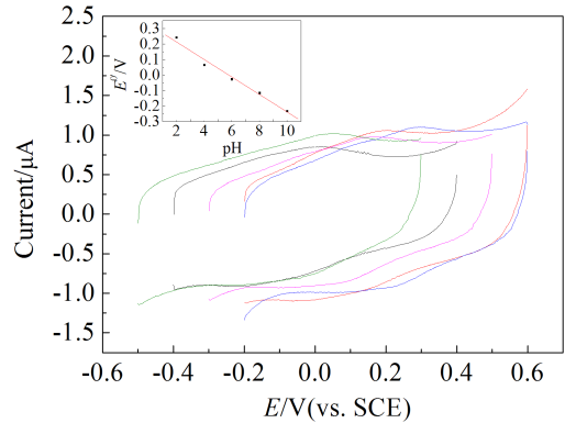
图 4 GOD/MspA-DMPC/GC 电极在 pH 2.00 (a)、4.00 (b)、6.00 (c)、8.00 (d) 和 10.00 (e) 0.1 mmol·L -1 PBS 缓冲溶液中的循环伏安曲线, 扫描速率: 200 mV·s -1 . 插图: 式量电位 ( E^0 ) 与 pH 的关系
