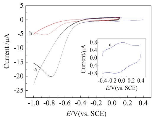
图 5 GOD/MspA-DMPC/GC 电极在被氧气饱 (a)、空气饱和 (b) 以及氮气饱和 (c) 0.1 mmol·L -1 PBS (pH 7.0) 缓冲溶液中的循环伏安曲线
