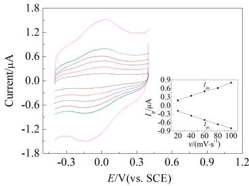
图 3 GOD/MspA-DMPC/GC 电极在 0.1 mmol·L -1 磷酸盐 (PBS) 缓冲溶液 (pH 7.0) 中的循环伏安曲线, 扫描速率 20~200 mV·s -1 (由内而外). 插图: 扫描速率 20~100 mV·s -1 时, 氧化峰电流 ( I_{pa} ) 和还原峰电流 ( I_{pc} ) 与扫描速率 ( v ) 的关系
