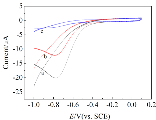
图 6 GOD/MspA-DMPC/GC 电极在氧气饱和和 0(a)、4.55 (b) 和 8.33 mmol·L -1 (c) 葡萄糖的 0.1 mmol·L -1 PBS(pH 7.0) 缓冲溶液中的循环伏安曲线
