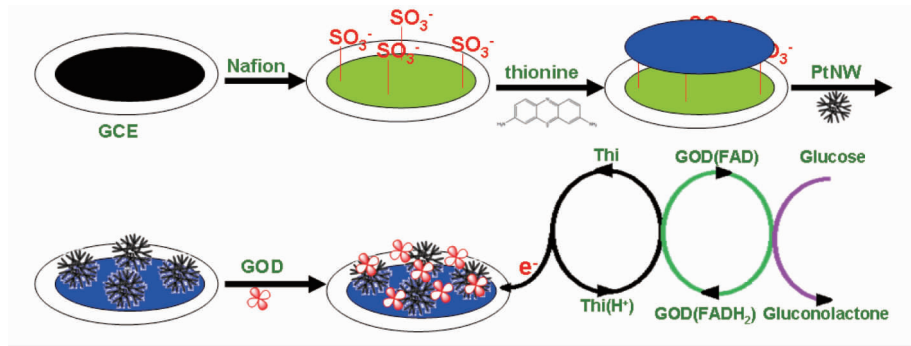
图 1 GOD/PtNW/Thi/Nafion/GC 电极及葡萄糖氧化机理的示意图
