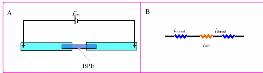
图 2 闭合式双极电极工作原理 A. 闭合式双极电极示意图;B. 等效电路图
