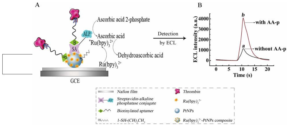
图 6 AA 与 Ru(bpy)_3^{2+} 共反应电致化学发光适体传感器电极的制备(A)及其催化性能(B) [28]
