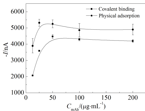
图 2 化学偶联或物理吸附组装不同浓度捕获探针对接流信号的影响 测试电位: -100 mV
