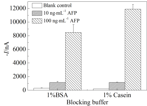
图 3 不同封闭液封闭电极后对检测 AFP 的响应电流信号的影响 测试电位: -100 mV
