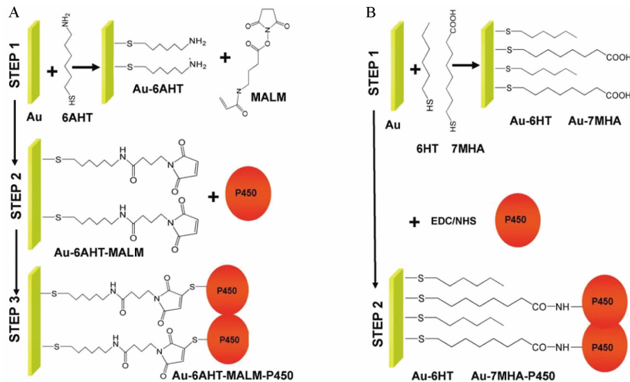
图 4 A. 金电极表面三步修饰 CYP2D6:1)6-氨基己硫醇(6AHT);2)与 3-马来酰亚胺基丙酸羧基琥珀酰亚胺酯(MALM)反应引入马来酰亚胺;3)马来酰亚胺与 CYP450 酶表面的氨基直接反应;B. 在金电极表面两步修饰 CYP2C9:1)6-己硫醇和 7-巯基庚酸(1:1)的 SAM 层;2)通过 1-乙基-3-(3-二甲氨基氨基丙基)碳化二亚胺盐酸化物(EDC)/N-羟基琥珀酰亚胺(NHS)作用下羧基与 CYP450 酶表面的氨基交联 [28]
