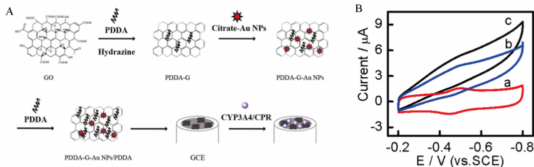
图 3 A. CYP3A4 传感器的构建; B. CYP3A4/CPR-microsomes/PDDA/Au/PDDA/G/GCE 在 0.1 \text{ mol}\cdot\text{L}^{-1} pH 7.4 PBS 溶液, 扫速 100 \text{ mV}\cdot\text{s}^{-1} 的循环伏安图(a. 无氧条件; b. 饱和空气; c. 含有饱和空气的 46 \mu\text{mol}\cdot\text{L}^{-1} 硝苯地平缓冲溶液) [20]
