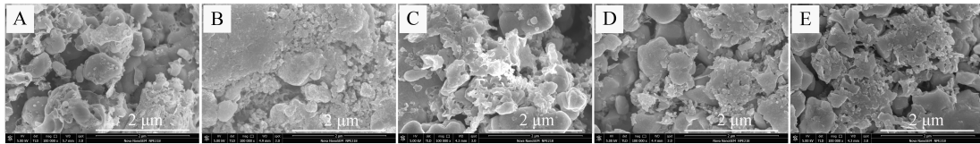
图 6 不同水分含量电池循环 200 周后正极 SEM 照片
