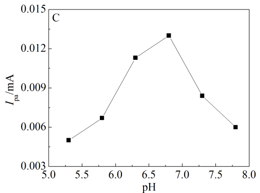
图 6 Pd/石墨烯/GCE 在不同 pH 的 CV 曲线 (A), pH 与 E_{pa} 的关系 (B), pH 与 I_{pa} 的关系 (C) 图 (PBS 支持电解质浓度 0.1 \text{ mol} \cdot \text{L}^{-1} , 4-氯酚浓度 100 \mu\text{mol} \cdot \text{L}^{-1} , 扫描速率 50 \text{ mV} \cdot \text{s}^{-1} )
