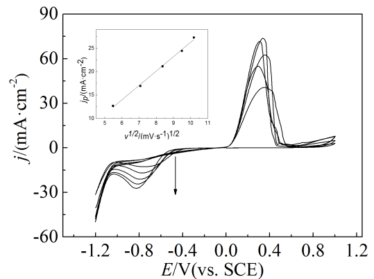
图1 不同扫描速率下银在玻碳电极表面沉积的循环伏安曲线
