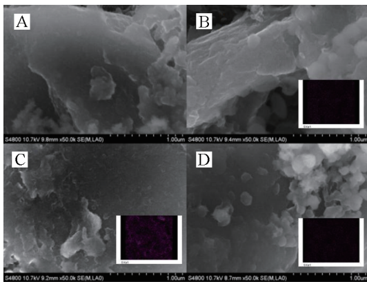
图 9 首周循环后的石墨表面 SEM 照片:
