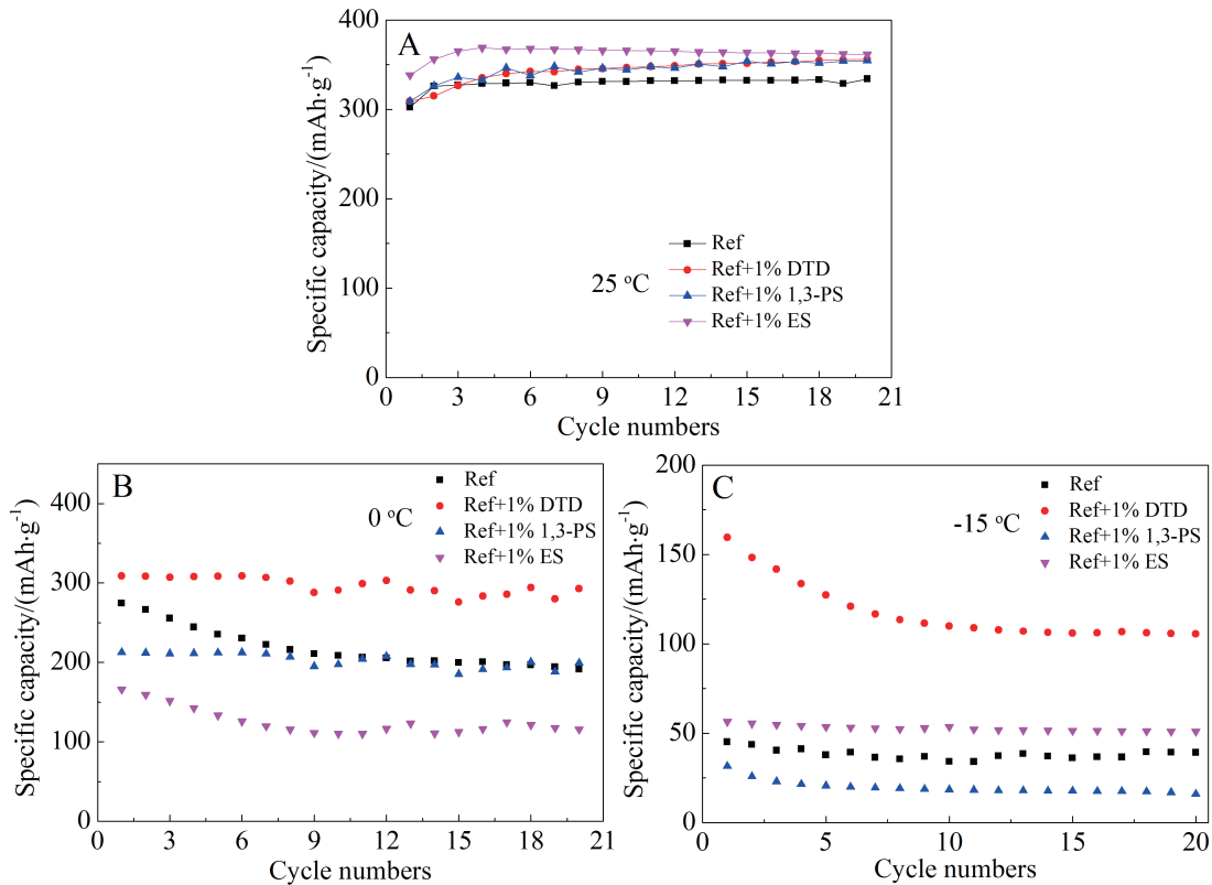
图 7 具有不同电解液组分的 AG/Li 电池在不同温度下的循环容量图
