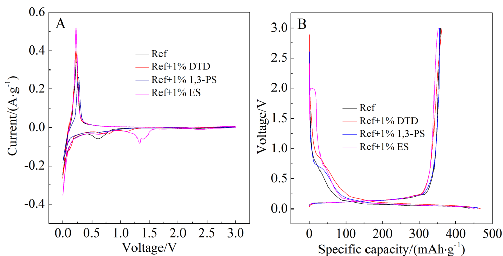
图 3 四组不同电解液的 AG/Li 电池的首周 CV 曲线, 扫速为 0.1 \text{ mV}\cdot\text{s}^{-1} (A) 和首周充放电曲线, 充放电倍率为 0.1C, 1\text{C} = 170 \text{ mAh}\cdot\text{g}^{-1} (B)
