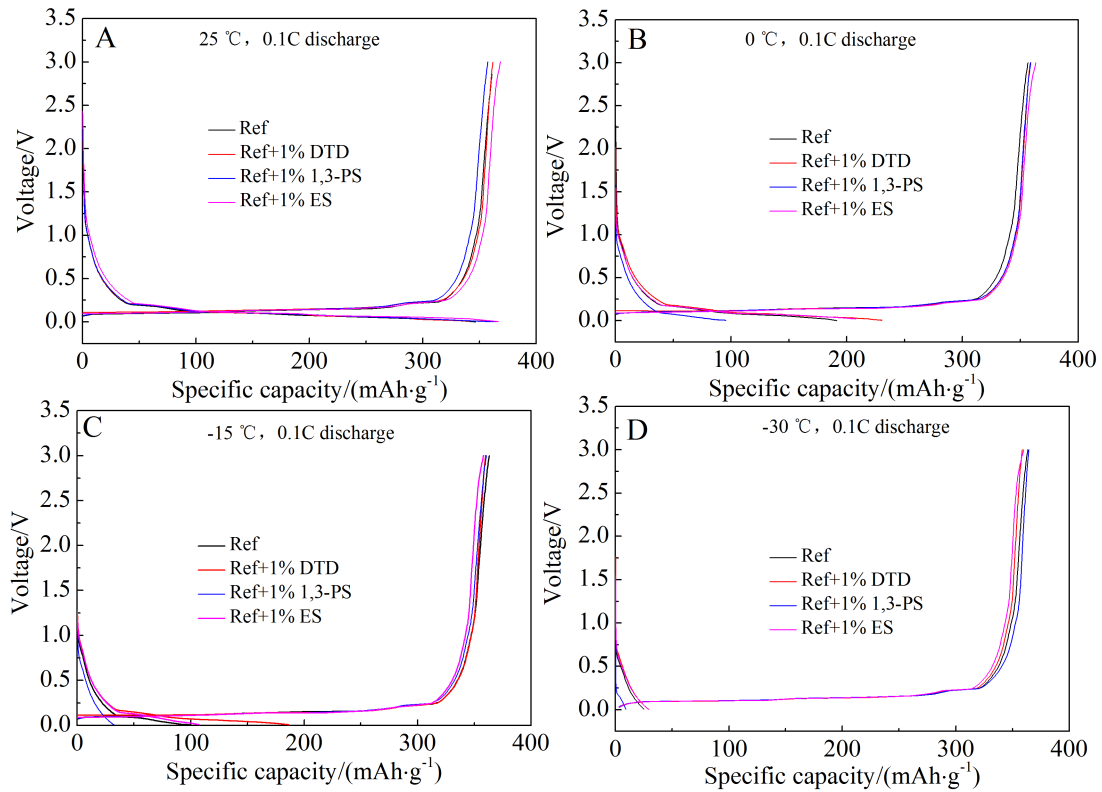
图 5 AG/Li 半电池在室温下充电、不同温度下放电的电化学曲线
