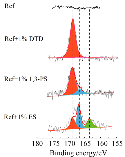
图 10 常温化成后的 AG 表面的 S2p 谱图
