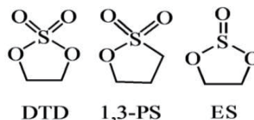
图 1 DTD、1,3-PS 和 ES 的结构式
