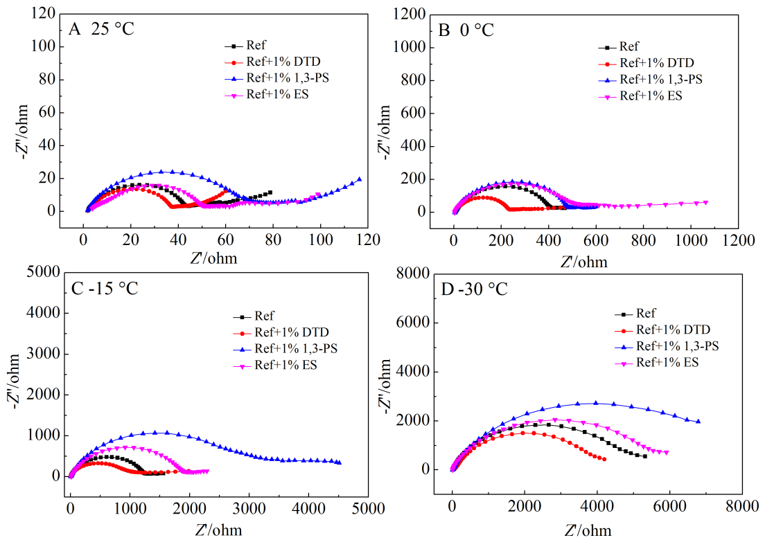
图 8 不同电解液组分的 AG/Li 电池在不同温度下的 EIS 曲线
