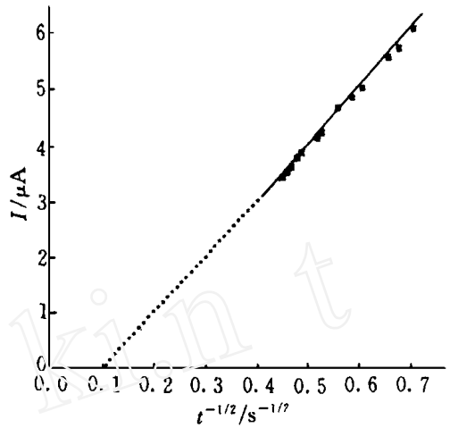
图 3 \text{Li}^+/\text{Sn}(\text{HPO}_4)_2 体系电位阶跃 I - t^{-1/2} 曲线(放电深度 x = 0.19 , 室温)
