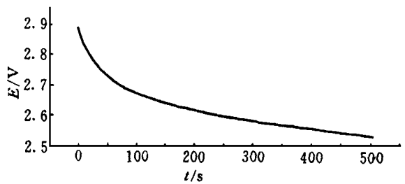
图 4 \text{Li}^+/\text{Sn}(\text{HPO}_4)_2 体系电流阶跃 V - t 图( I = 0.5\ \mu\text{A} , x = 0.19 , 室温)
