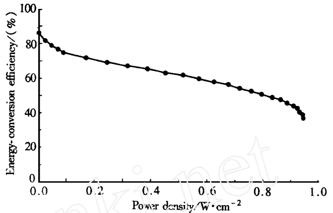
图 5 Nafion 112 膜和 E-TEK 电极组装的 PEMFC 能量转换效率与功率密度变化曲线
