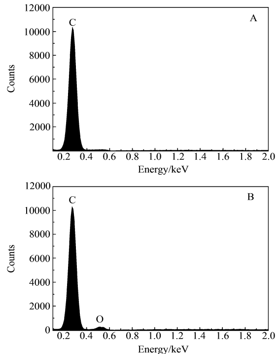
图 3 不同时间氧气等离子体处理石墨基底的 EDS 谱图 A. 0 min; B. 15 min
