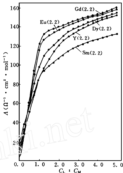
图 2 25 °C 在 (\text{CH}_3)_2\text{CO} 溶液中穴醚 (2.2) 对 (\text{NO}_3)_3 电导滴定曲线
