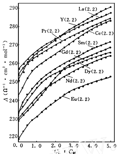
图 1 25 °C 在 DMF 溶液中穴醚 (2.2) 对 \text{Ln}(\text{NO}_3)_3 电导滴定曲线
